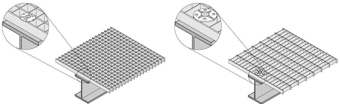
Sicherung quadratischer Gitterroste
